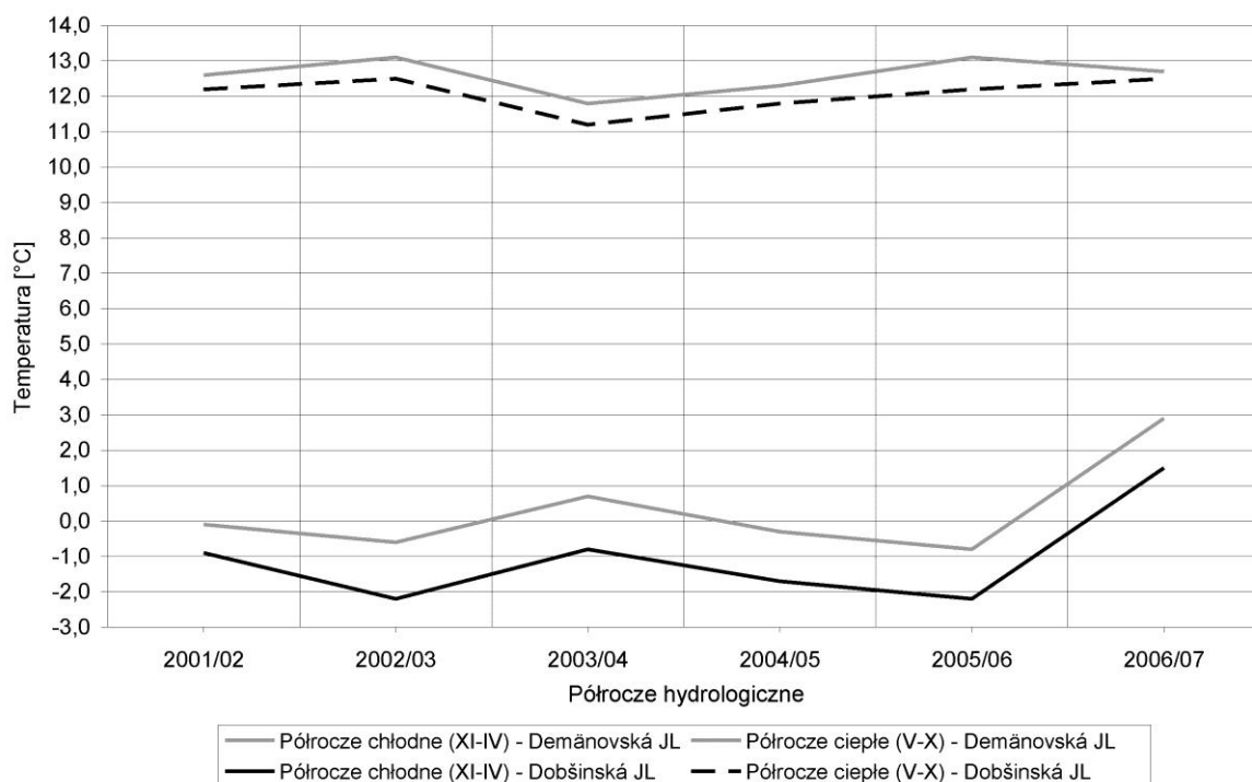
Ryc. 43. Przebieg temperatury powietrza w otoczeniu Demänovskiej JL i Dobšinskéj JL w okresie od 2001/02 do 2006/07; wg średnich wielkości z półrocza chłodnego i półrocza ciepłego (opracowanie własne).
