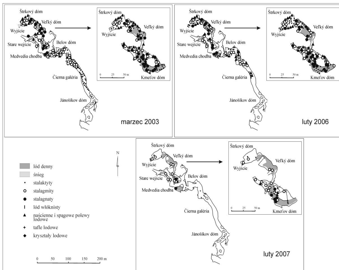
Ryc. 104. Rozmieszczenie i typy form lodowych w Demänovskiej JL w marcu 2003, w lutym 2006 oraz w lutym 2007 roku; w prawych górnych rogach formy lodowe w zalodzionym fragmencie jaskini (opracowanie własne).
