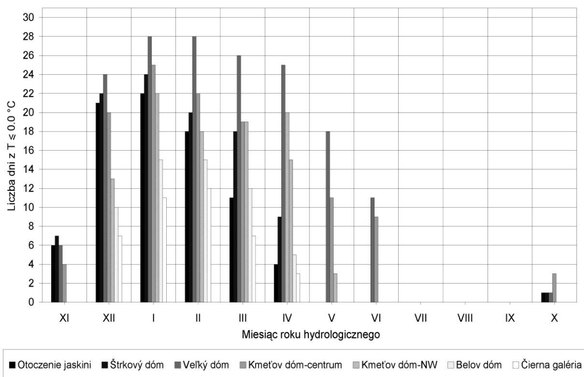
Ryc. 58. Przeciętna liczba dni z temperaturą powietrza mniejszą lub równą 0,0°C w miesiącu w otoczeniu oraz w poszczególnych komorach Demänovskiej JL; wg uśrednionych wielkości dobowych z okresu 2001/02–2006/07 (opracowanie własne).
