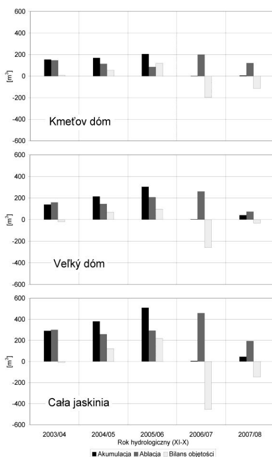
Ryc. 83. Roczna akumulacja, ablacja oraz bilans objętości lodu dennego (w m 3 ) w komorze Kmeťov dóm i Veľký dóm oraz w całym zalodzionym fragmencie Demänovskiej JL w okresie od 2003/04 do 2007/08 (opracowanie własne na podstawie: Strug, Zelinka 2008b).
