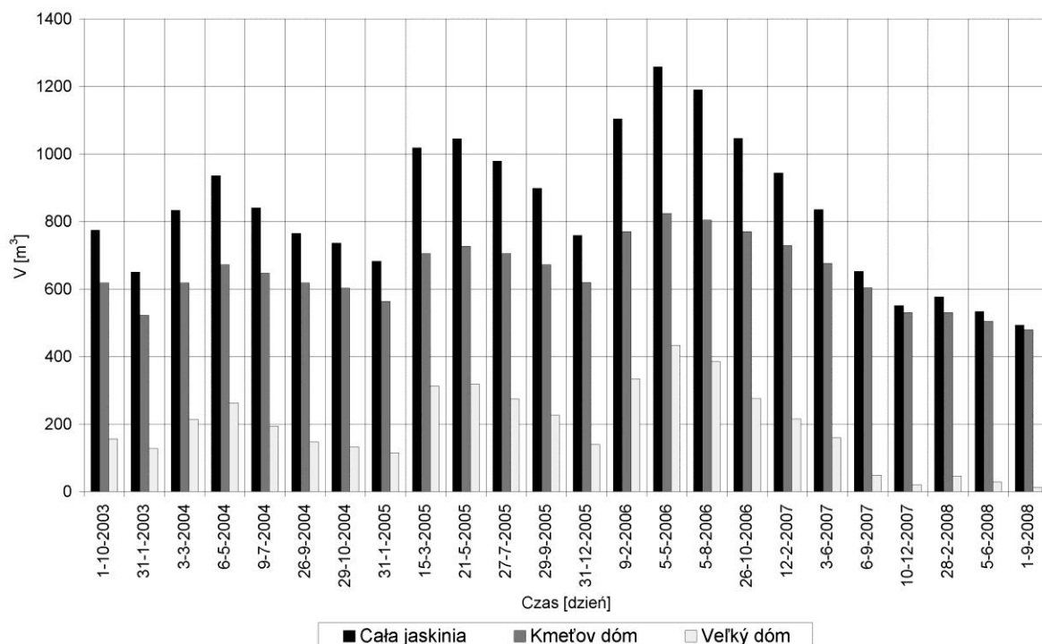
Ryc. 81. Zmiany objętości ( V ) lodu dennego w komorze Kmet'ov dóm i Velký dóm oraz w całym zalodzonej fragmencie Demänovskiej JL w okresie od 01.10.2003 do 01.09.2008 (opracowanie własne na podstawie: Strug, Zelinka 2008b).
