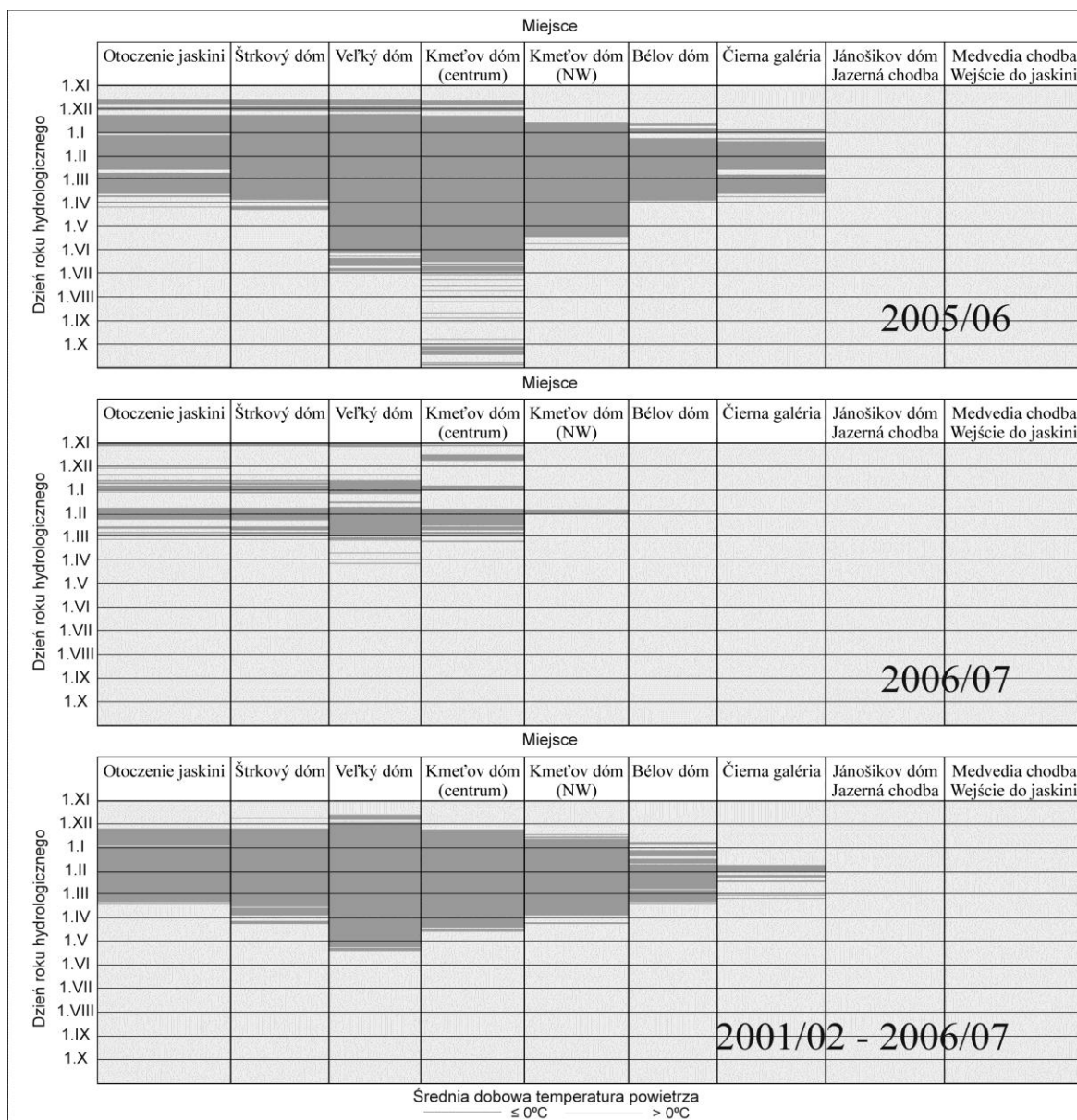
Ryc. 56. Występowanie dni z temperaturą powietrza mniejszą lub równą 0.0^{\circ}\text{C} i większą od 0.0^{\circ}\text{C} w otoczeniu oraz w poszczególnych komorach Demänovskiej JL w roku hydrologicznym 2005/06 i 2006/07 oraz przeciętne występowanie tych dni w okresie 2001/02-2006/07 (opracowanie: Strug, Zelinka 2008a).
