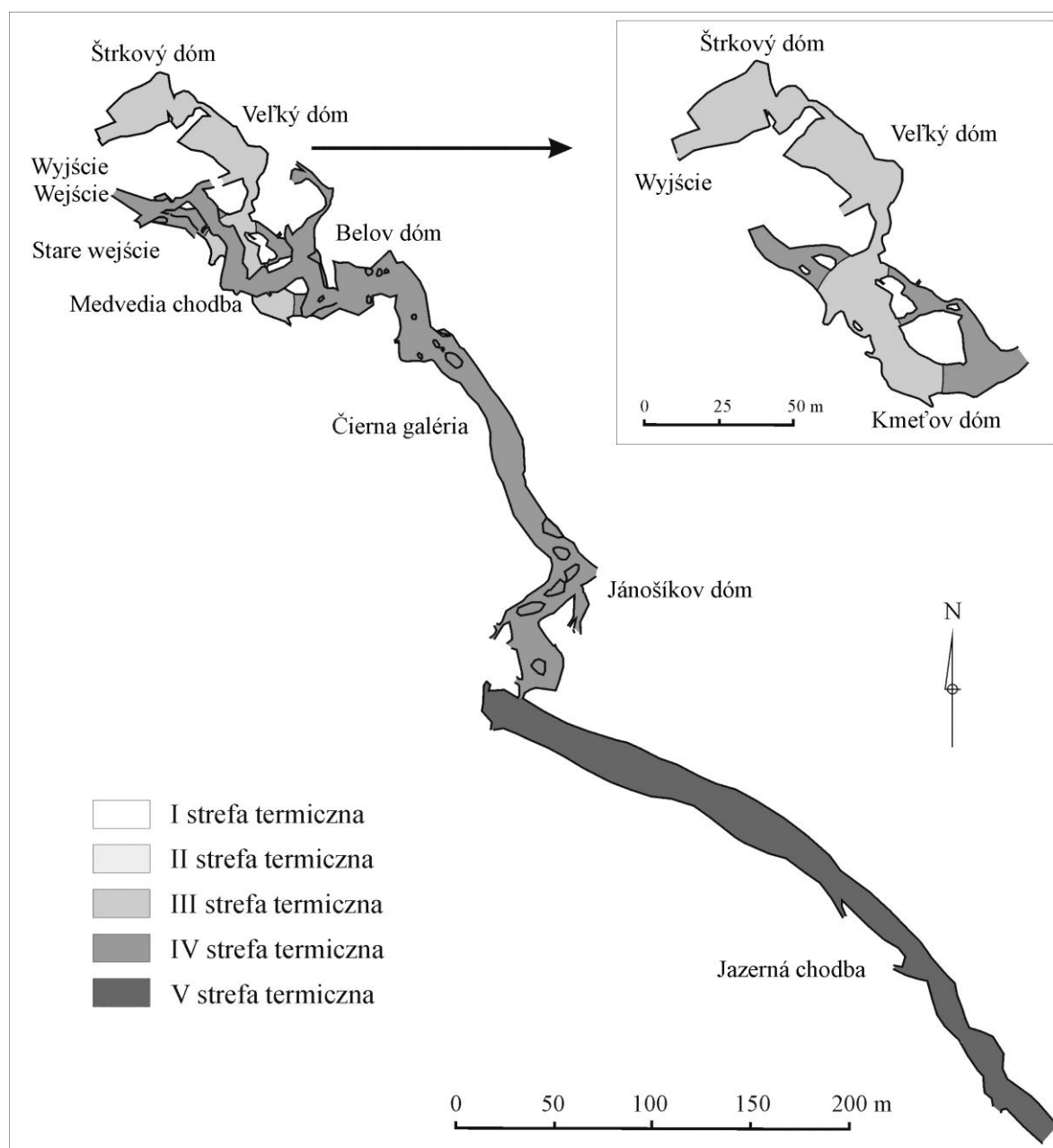
Ryc. 71. Zasięg występowania stref termicznych w Demänovskej JL w roku hydrologicznym 2006/07; w prawym górnym rogu zasięg stref w zalodonym fragmencie jaskini (opracowanie własne na podstawie: Piasecki i in. 2007).
