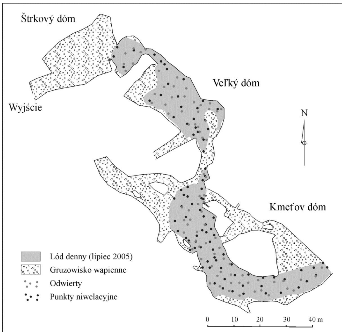
Ryc. 22. Lokalizacja odwiertów i punktów niwelacyjnych w zalodzonym fragmencie Demänovskej JL (opracowanie: Strug i in. 2006).
