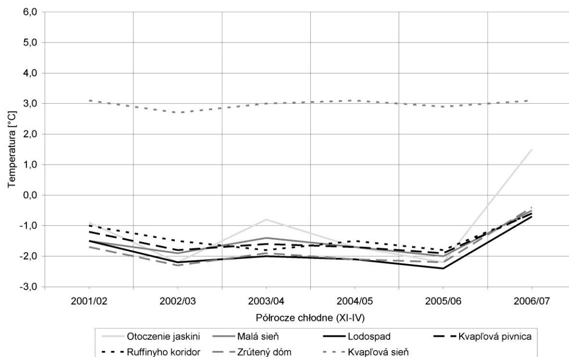
Ryc. 47. Przebieg temperatury powietrza w otoczeniu oraz w poszczególnych komorach Dobšinskiej JL w okresie od 2001/02 do 2006/07; wg średnich wielkości z półrocza chłodnego (opracowanie własne).
