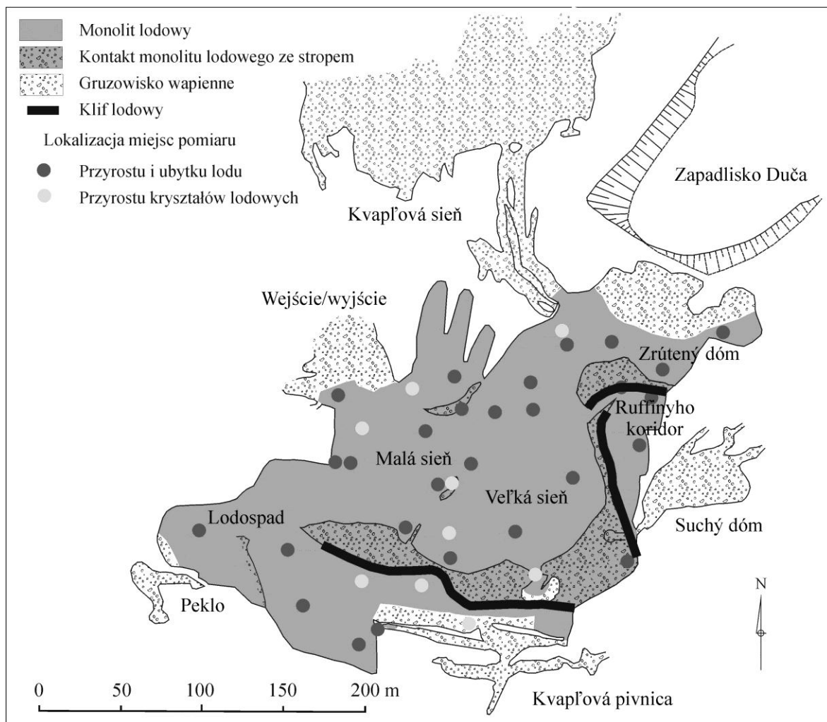
Ryc. 25. Lokalizacja miejsc pomiaru przyrostu i ubytku lodu oraz przyrostu kryształów lodowych w Dobšinskiej JL (opracowanie własne).
