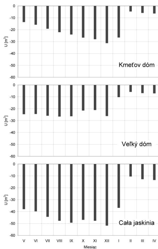
Ryc. 86. Przeciętny roczny ubytek (U) lodu dennego w komorze Kmeťov dóm i Veľký dóm oraz w całym zalodzionym fragmencie Demänovskiej JL; wg uśrednionych wielkości miesięcznych z okresu 2003/04-2007/08 (opracowanie własne).
