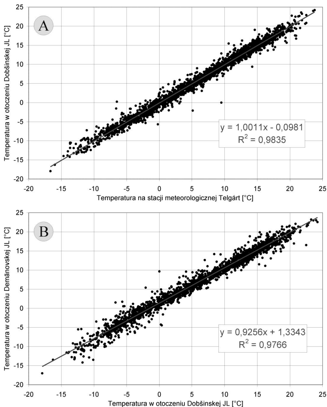
Ryc. 31. Średnia dobową temperaturę powietrza w otoczeniu Dobšinskiej JL względem stacji meteorologicznej Telgárt (A) oraz w otoczeniu Demänovskiej JL względem otoczenia Dobšinskiej JL (B) w okresie 2001/02-2006/07 (opracowanie własne).
