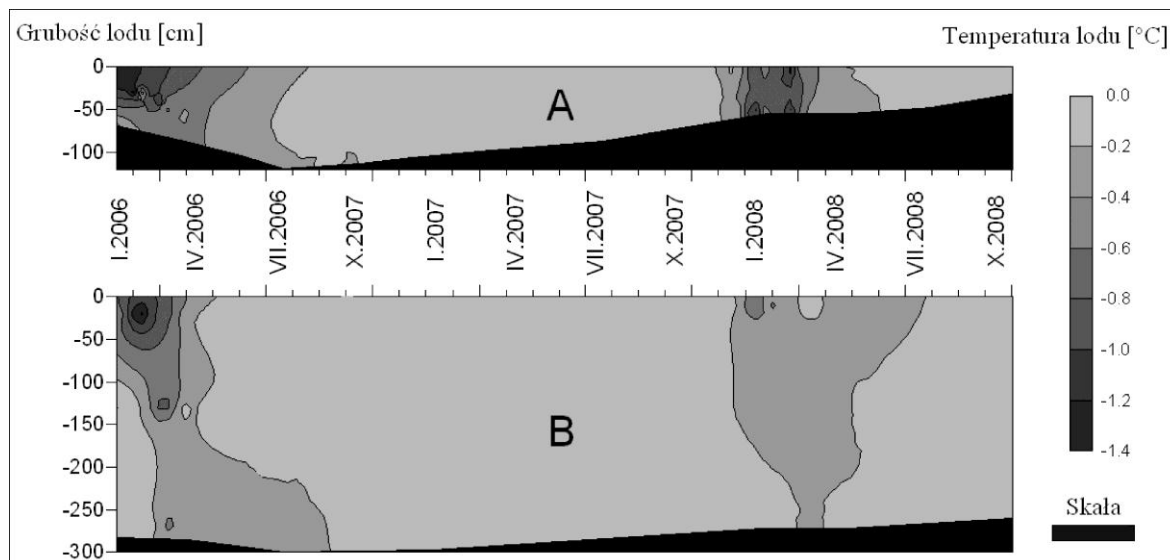
Ryc. 76. Przebieg temperatury lodu dennego w Demänovskej JL w komorze Veľký dom (punkt A) i Kmeťov dom (punkt B) w okresie od stycznia 2006 do października 2008 roku (opracowanie własne na podstawie: Strug, Zelinka 2008c).
