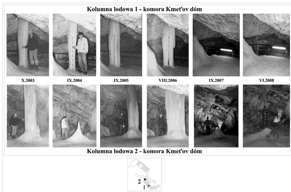
Ryc. 106. Rozmiary wybranych kolumn lodowych w Demänovskej JL pod koniec roku hydrologicznego w okresie od 2002/03 do 2007/08 (opracowanie własne; fot: T. Sawiński, K. Strug, R. Szmytkie, za zgodą autorów).
