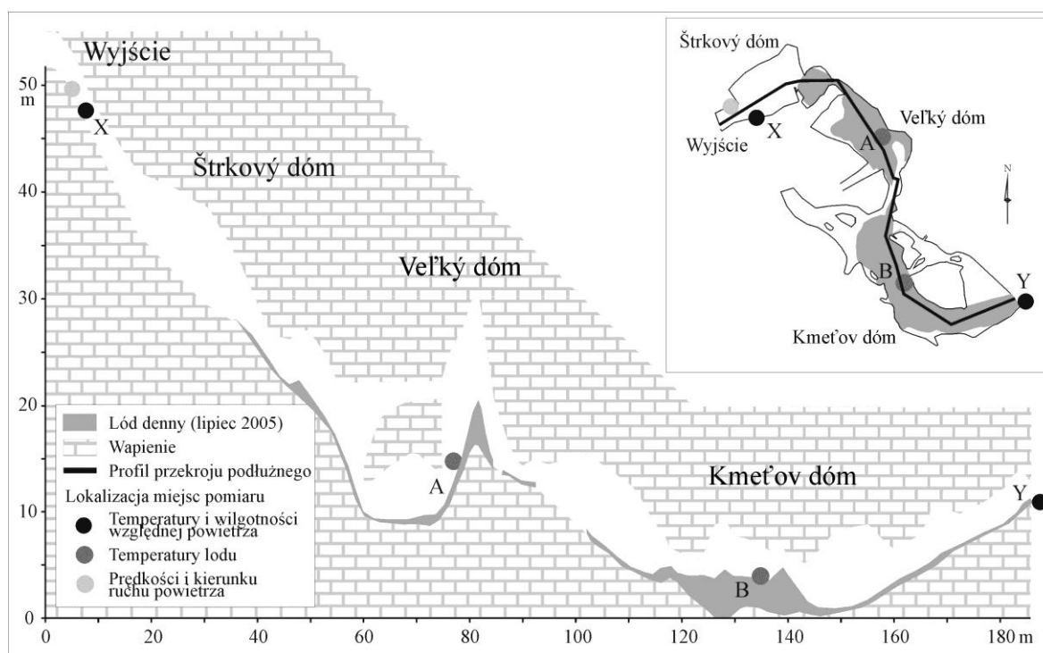
Ryc. 33. Lokalizacja miejsc pomiaru temperatury, prędkości i kierunku ruchu powietrza oraz wilgotności względnej w zalodzionym fragmencie Demänovskiej JL – przekrój podłużny i plan (opracowanie: Strug i in. 2008b).
