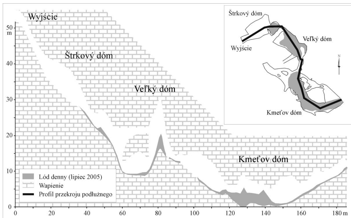
Ryc. 8. Zalodzony fragment Demänovskej JL – przekrój podłużny i plan (opracowanie: Strug i in. 2008b).
