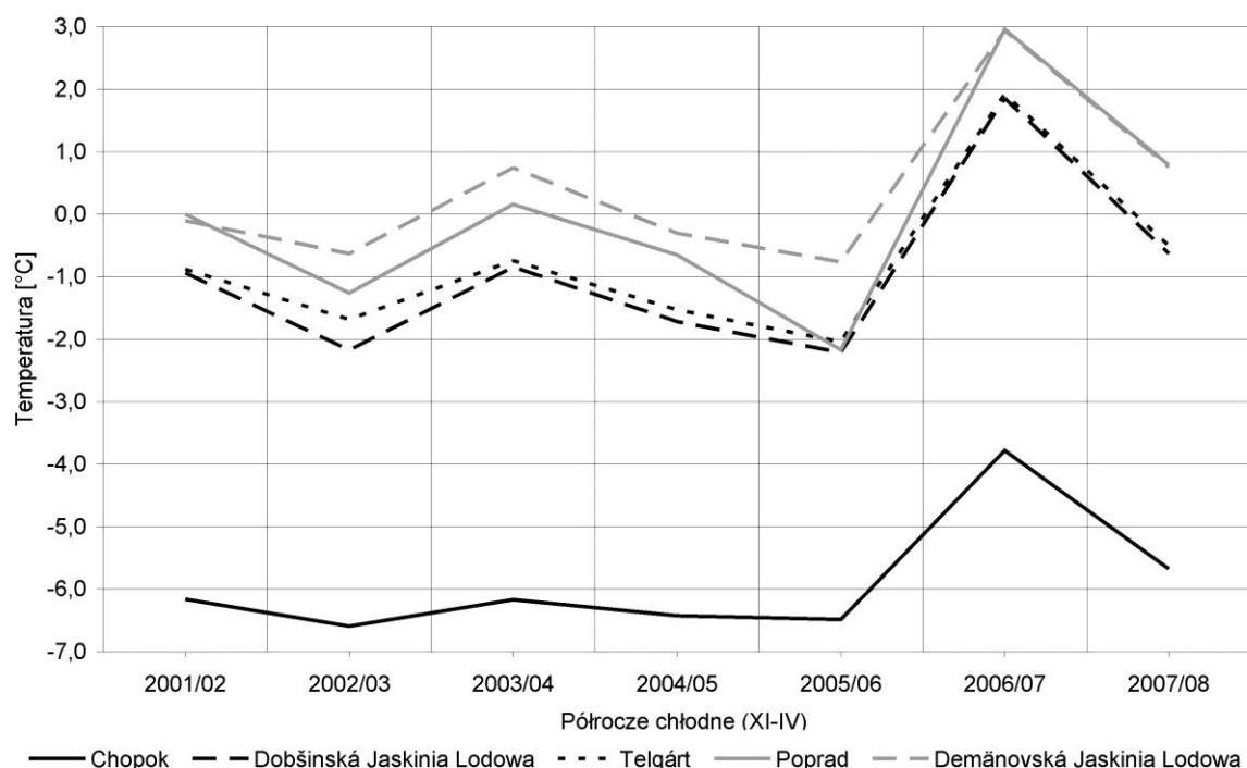
Ryc. 44. Przebieg temperatury powietrza na stacji meteorologicznej Chopok, Telgárt i Poprad oraz w otoczeniu Demänovskiej JL i Dobšinskéj JL w okresie od 2001/02 do 2007/08; wg średnich wielkości z półrocza chłodnego (opracowanie własne na podstawie: Strug, Zelinka 2008c).
