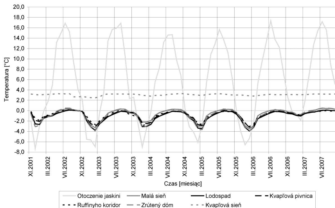
Ryc. 49. Przebieg temperatury powietrza w otoczeniu oraz w poszczególnych komorach Dobšinskej JL w okresie od listopada 2001 do października 2007 roku; wg średnich wielkości miesięcznych (opracowanie własne).
