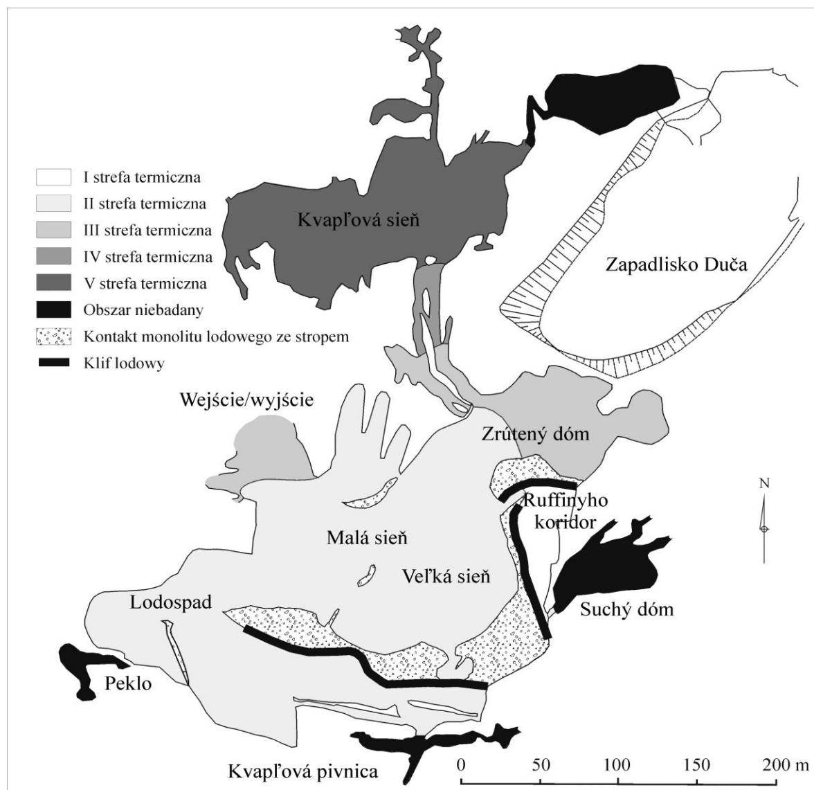
Ryc. 72. Zasięg występowania stref termicznych w Dobšinskiej JL w roku hydrologicznym 2006/07 (opracowanie własne).
