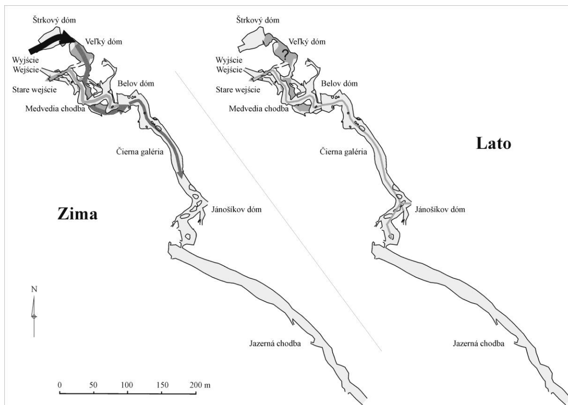
Ryc. 40. Schemat cyrkulacji powietrza w zimie i lecie w Demänovskej JL (opracowanie własne na podstawie: Piasecki i in. 2007, Strug i in. 2008b).
