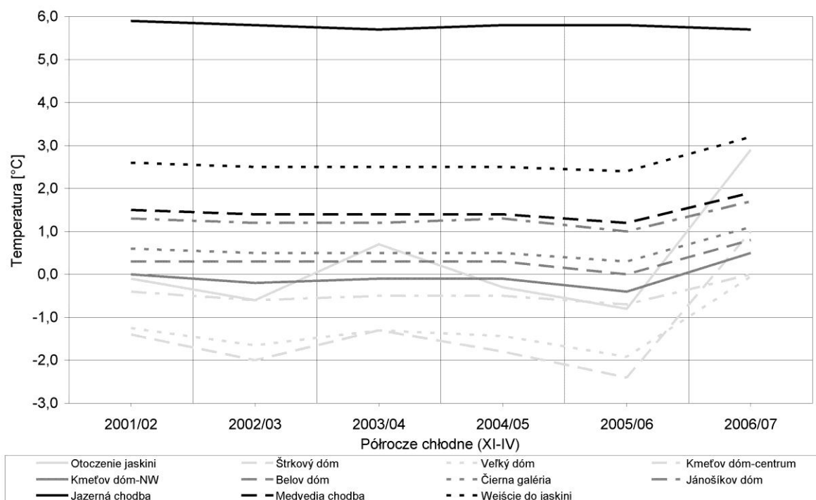
Ryc. 46. Przebieg temperatury powietrza w otoczeniu oraz w poszczególnych komorach Demänovskiej JL w okresie od 2001/02 do 2006/07; wg średnich wielkości z półrocza chłodnego (opracowanie własne).
