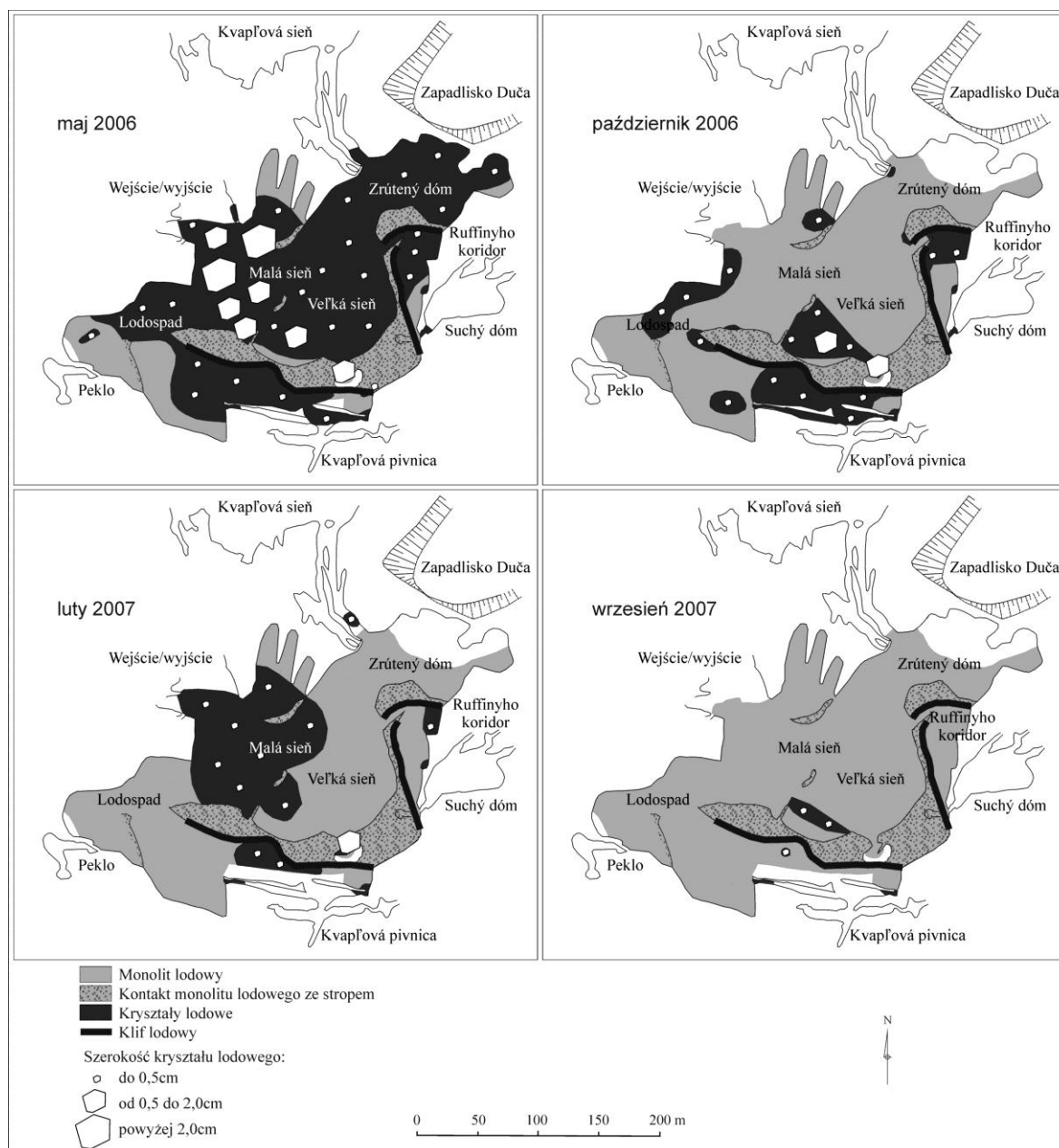
Ryc. 103. Maksymalny i minimalny zanotowany zasięg występowania kryształów lodowych w Dobšinskéj JL w roku hydrologicznym 2005/06 i 2006/07; w trzech klasach ich szerokości (opracowanie: Strug, Zelinka 2008c).
