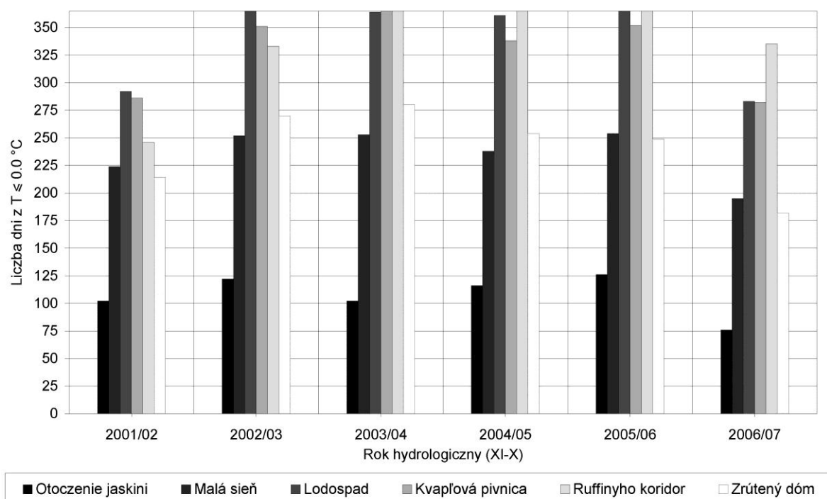
Ryc. 55. Liczba dni z temperaturą powietrza mniejszą lub równą 0.0^\circ\text{C} w roku hydrologicznym w otoczeniu oraz w poszczególnych komorach Dobšinskéj JL w okresie od 2001/02 do 2006/07; wg średnich wielkości dobowych (opracowanie własne).
