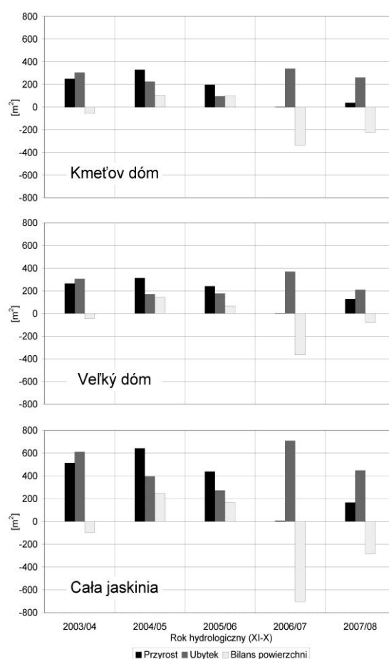
Ryc. 84. Roczny przyrost, ubytek oraz bilans powierzchni lodu dennego (w m 2 ) w komorze Kmeťov dóm i Veľký dóm oraz w całym zalodzionym fragmencie Demänovskiej JL w okresie od 2003/04 do 2007/08 (opracowanie własne na podstawie: Strug, Zelinka 2008b).
