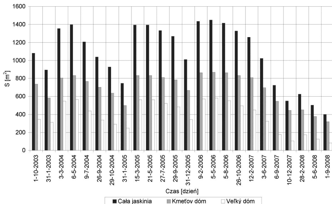
Ryc. 82. Zmiany powierzchni ( S ) lodu dennego w komorze Kmet'ov dóm i Velký dóm oraz w całym zalodzonej fragmencie Demänovskiej JL w okresie od 01.10.2003 do 01.09.2008 (opracowanie własne na podstawie: Strug, Zelinka 2008b).
