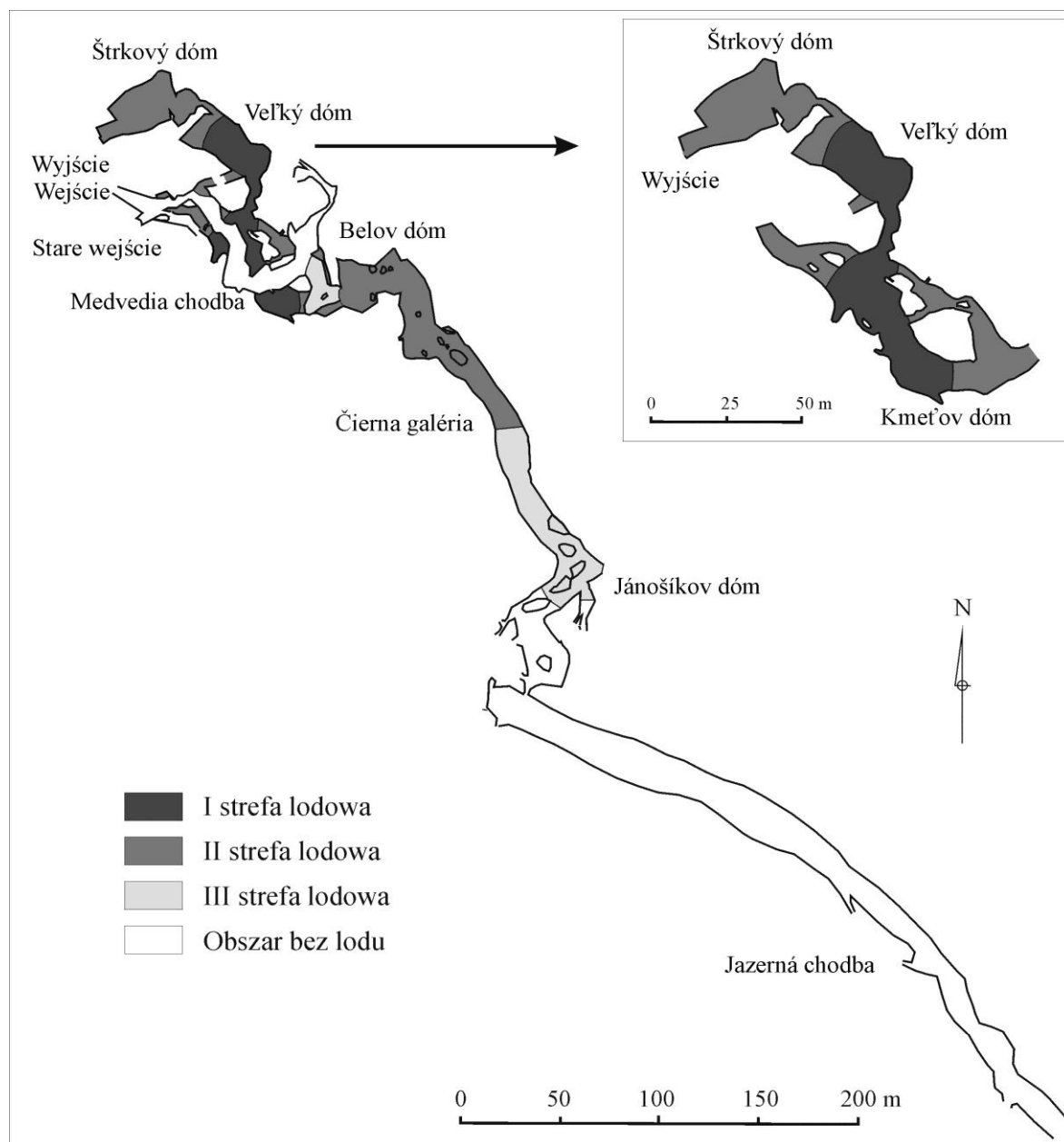
Ryc. 73. Przeciętny zasięg występowania stref lodowych oraz obszaru pozbawionego lodu w Demänovskej JL w okresie 2002/03–2007/08; w prawym górnym rogu zasięg stref w zalodzonej fragmentacji jaskini (opracowanie własne na podstawie: Piasecki i in. 2007).
