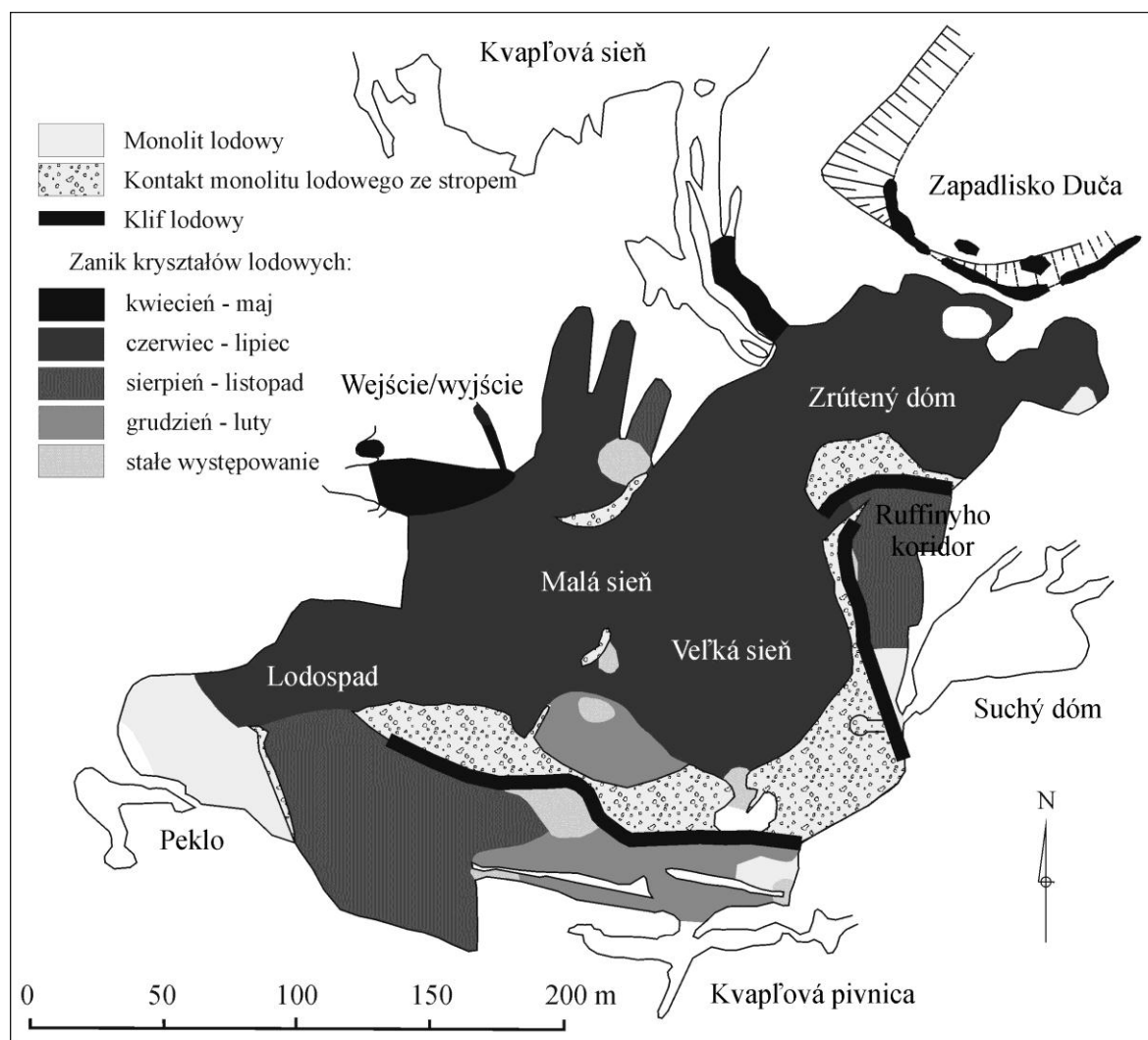
Ryc. 102. Przekiętny zanik (w miesiãcach) kryształów lodowych na stropie w Dobšinské JL; na podstawie obserwacji z okresu 2003-2008 (opracowanie: Piasecki i in. 2007).
