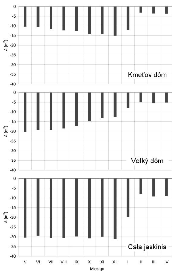
Ryc. 85. Przeciętna roczna ablacja (A) lodu dennego w komorze Kmeťov dóm i Veľký dóm oraz w całym zalodzionym fragmencie Demänovskiej JL; wg uśrednionych wielkości miesięcznych z okresu 2003/04-2007/08 (opracowanie własne).
