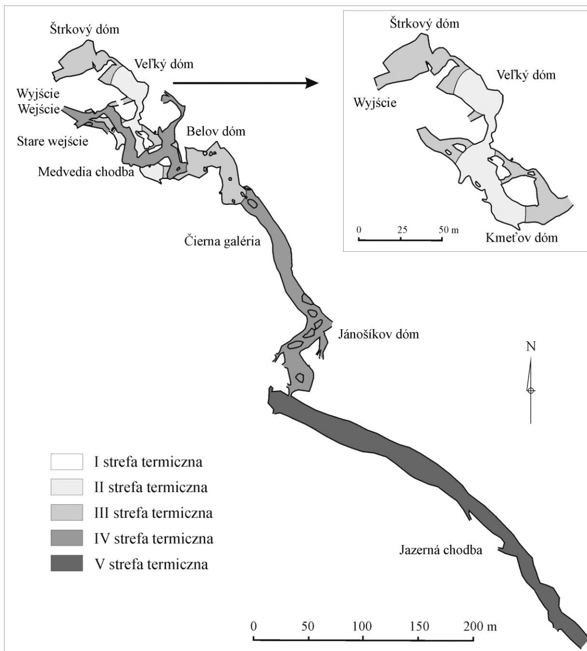
Ryc. 65. Przeciętny zasięg występowania stref termicznych w Demänovskiej JL w okresie 2001/02–2006/07; w prawym górnym rogu zasięg stref w zalodzonej fragmentacji jaskini (opracowanie własne na podstawie: Piasecki i in. 2007).
