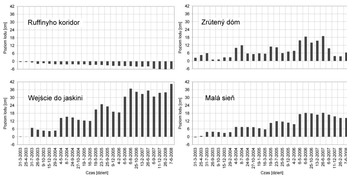
Ryc. 89. Zmiany poziomu monolitu lodowego w sali Malá sieň, w obszarze wejściowym do jaskini, w sali Zrútený dóm oraz w korytarzu Ruffinyho koridor w Dobšinskiej JL w okresie od 31.03.2003 do 07.06.2008 w stosunku do jego poziomu z dnia 24.02.2003 (opracowanie własne).
