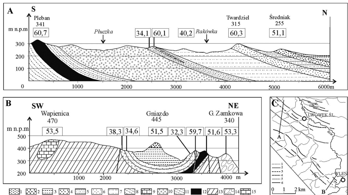
Ryc. 56. A i B – średni odbiór młotka Schmidta wzdłuż wybranych przekrojów we wschodniej części Pogórza Izerskiego; kenozoik: 1 – bazalty, górna kreda: 2 – piaskowce ciosowe koniak, 3 – margle koniak, 4 – piaskowce ciosowe turonu, 5 – piaskowce wapieniste i margle turonu, 6 – piaskowce ciosowe cenomanu, dolny trias: 7 – piaskowce kwarcowe cienkoławicowe, górny perm: 8 – łupki ilaste, 9 – wapień dolomityczny, dolny perm: 10 – zlepińce drobnoziarniste i piaskowce, 11 – łupki ilasto-piaszczyste, 12 – trachybazalty, dolny paleozoik: 13 – łupki kwarcowo-serycytowe, 14 – zieleńce i spillity, 15 – wapień krystaliczny. C – lokalizacja przekrojów na tle przebiegu krawędzi strukturalnych założonych na wychodniach: piaskowców ciosowych górnej kredy (1 – koniak, 2 – turonu, 3 – cenomanu) i dolnego triasu (4) oraz na wapieniach górnego permu (5) i trachybazaltach dolnego permu (6). Opracowanie własne na podstawie przekrojów geologicznych zamieszczonych na Szczegółowej Mapie Geologicznej Sudetów 1:25 000 w arkuszach Wleń i Lwówek Śląski
