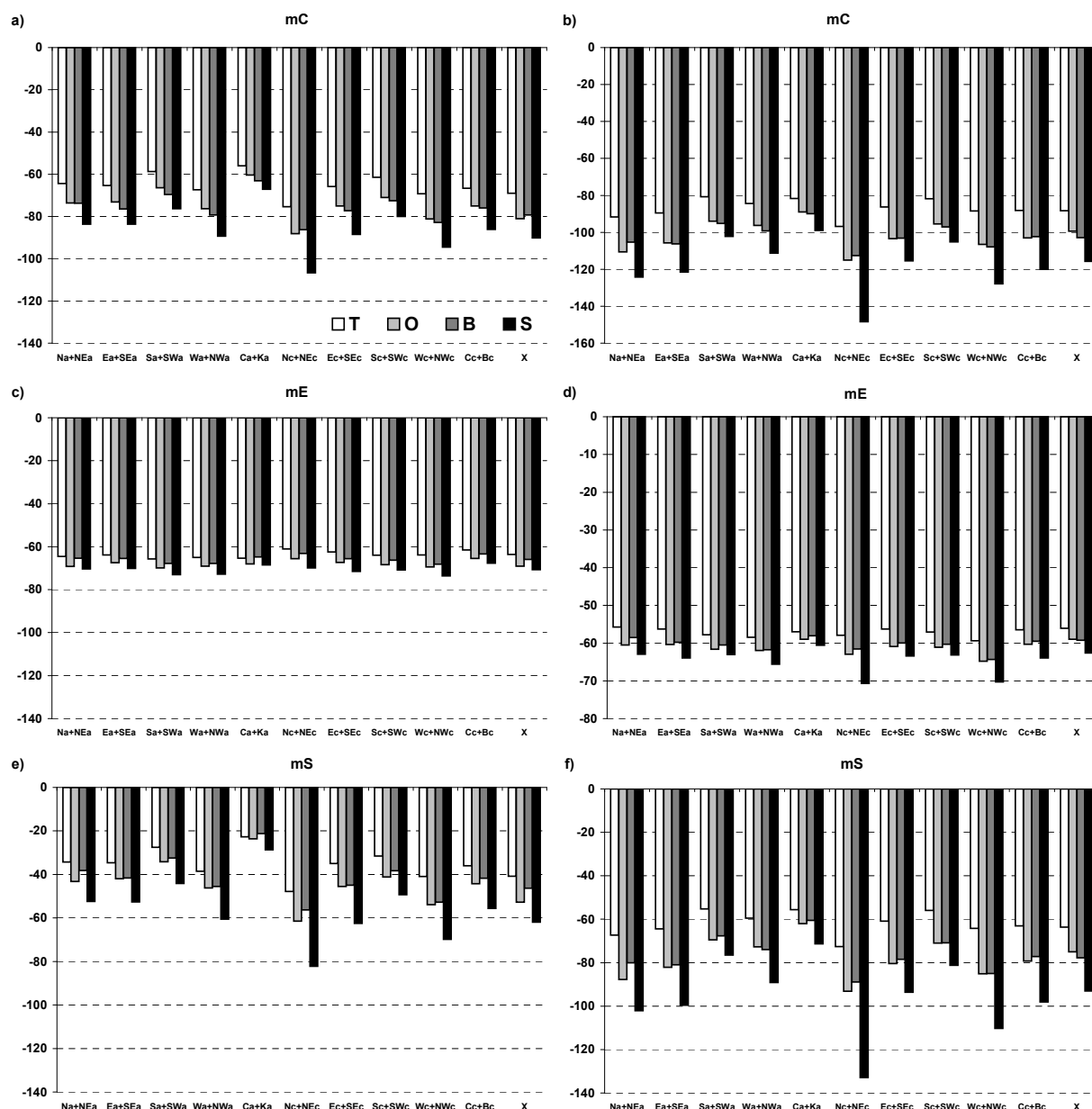
Ryc. 77. Średnie wartości strumienia konwekcyjnego ( mC , W/m^2 ) i ewaporacyjnego ( mE , W/m^2 ) wymiany ciepła między człowiekiem a otoczeniem oraz saldo ( mS , W/m^2 ) w określonych typach cyrkulacji (wg Niedźwiedzia) w półroczu ciepłym (a, c, e) i chłodnym (b, d, f) we Wrocławiu, IV 2001-VII 2004
