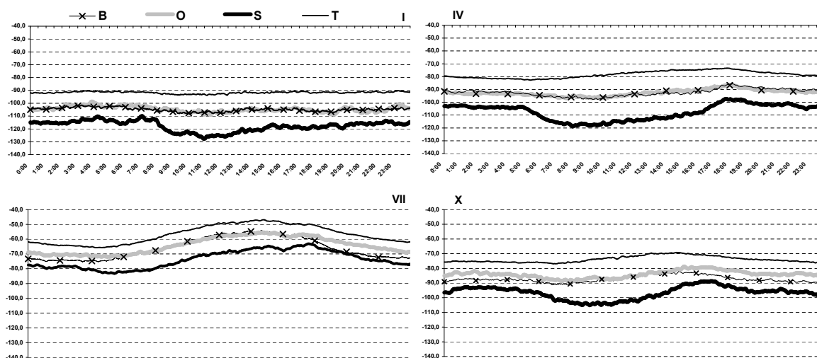
Ryc. 72. Średni dobowy przebieg wartości konwekcyjnego strumienia wymiany ciepła ( mC , W/m^2 ) w wybranych miesiącach (styczeń, kwiecień, lipiec i październik) w różnych typach zabudowy we Wrocławiu, IV 2001-VII 2004. Wartości średnie zostały „wygładzone” średnią konsekutywną 11-minutową
