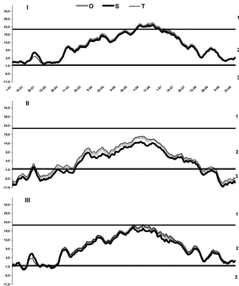
Ryc. 81. Roczny przebieg średnich wartości temperatury odczuwalnej ( T_c , °C) w daytime (I) i nocnej (II) porze doby oraz w ciągu całej doby (III) we Wrocławiu. Z prawej strony umieszczono skalę odczuć cieplnych: 1- zimno, 2- chłodno, 3- komfortowo, (wartości średnie dobowe zostały „wygładzone” średnią konsekwentną 11-dniową)
